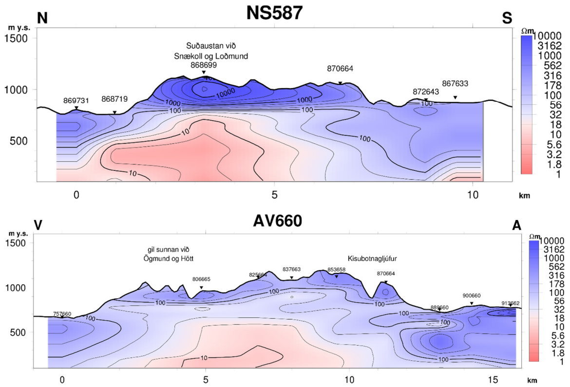
Mynd 4-3: Viðnámsnið af Kisubotnum (Ragna Karlsdóttir o.fl., 2010).
