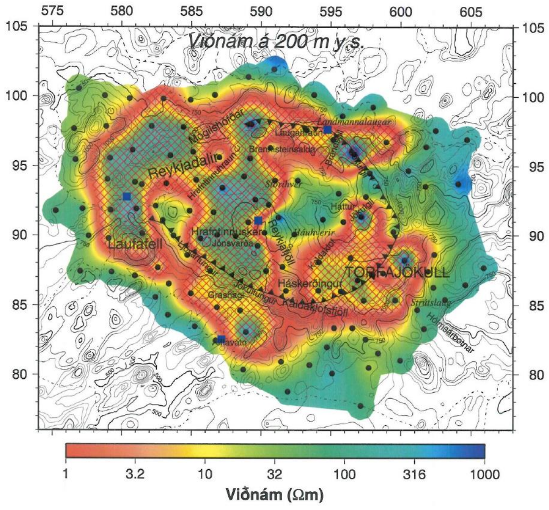
Mynd 4-6: Viðnámskort af svæðinu (skástrikuðu svæðin tákna háviðnámskjarna) (Ragna Karlsdóttir, 2003).
