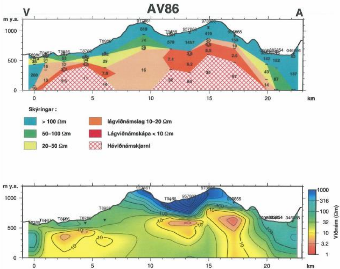
Mynd 4-7: Viðnámssnið af Sandfellssvæðinu (Ragna Karlsdóttir, 2003).
