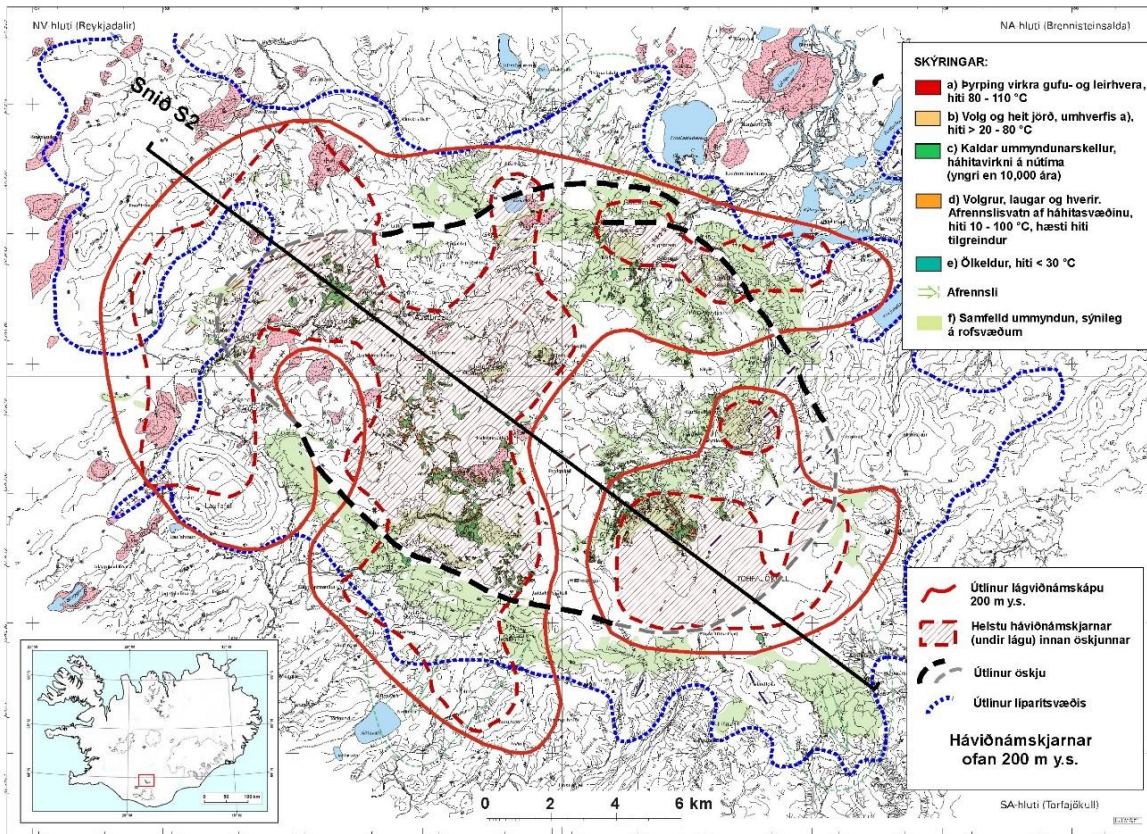
Mynd 4-3: Lágviðnámskápa og háviðnámskjarni á Torfajökullssvæðinu (Jónas Ketilsson o.fl., 2010).
