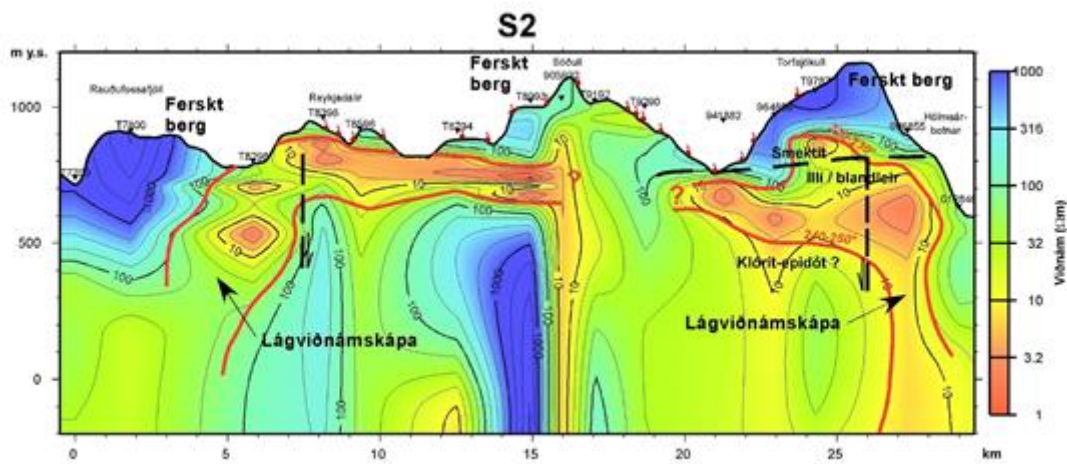
Mynd 4-4: Viðnámsþversnið af Torfajökullssvæðinu (Jónas Ketilsson o.fl., 2010).
